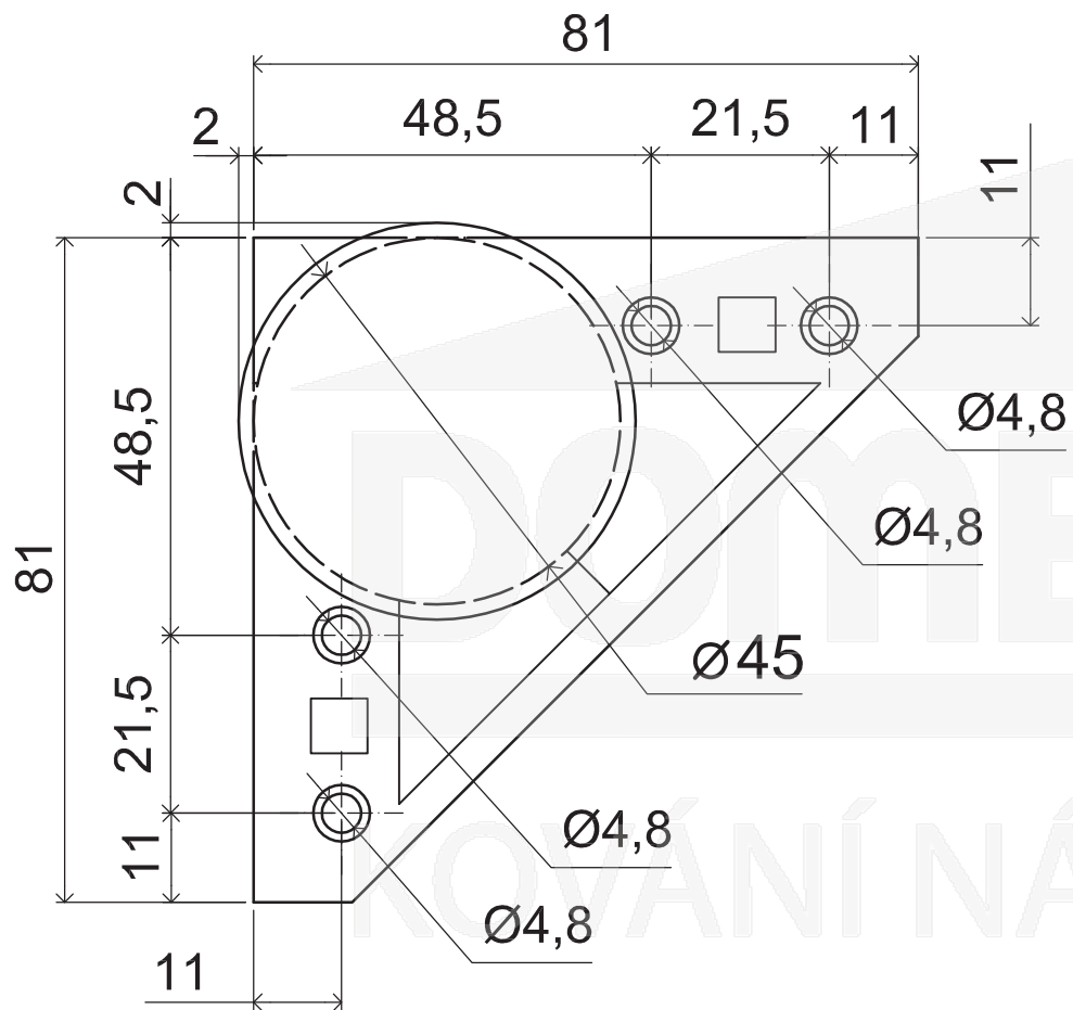
Pohled na montážní plotnu zespodu
