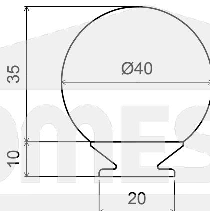
typ krčku B
