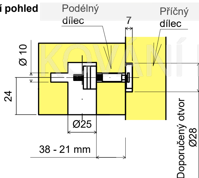
Horní pohled
