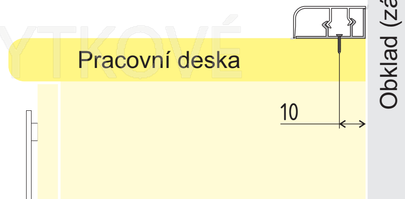
Ohebné těsnění
